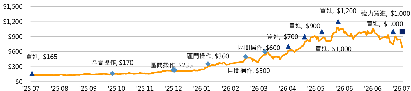
歷史投資建議走勢
